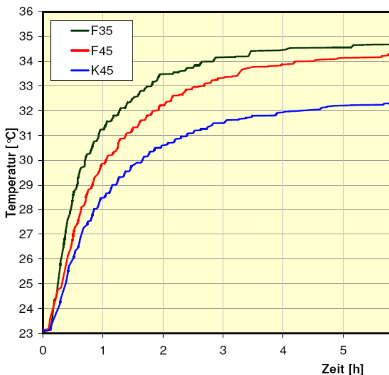
Entwicklung der Oberflächentemperatur an Estrichproben
