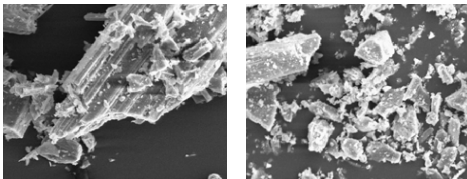
Abb. 9: REM-Aufnahmen von Alpha-Halbhydrat in einem handelsüblichen Fließestrich
