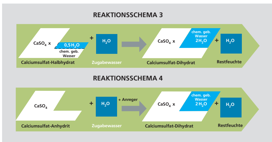
Abb. 2: Die Rückbildung (Festigkeitsbildung) von Calciumsulfat-Dihydrat aus Calciumsulfat-Halbhdydrat (3) und Calciumsulfat-Anhydrit (4)
