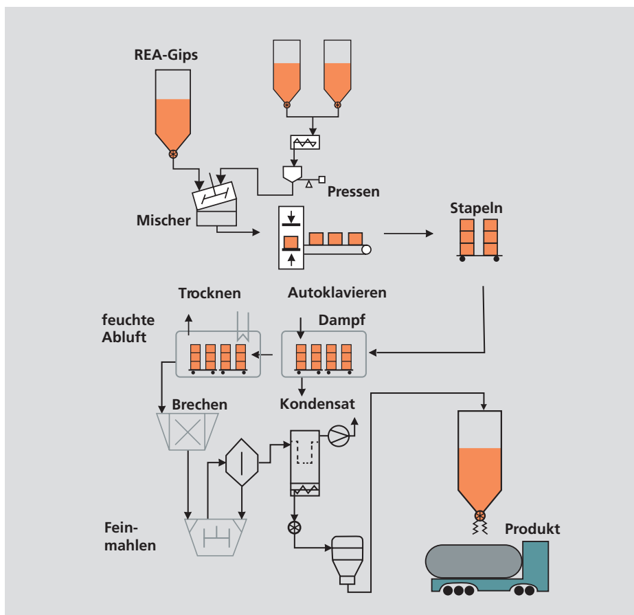
Abb. 8: Die Bildung von Calciumsulfat-Alpha-Halbhydrat aus REA-Gips
