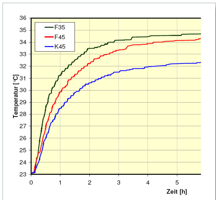
Abb.1: Entwicklung der Oberflächentemperatur an Estrichproben
