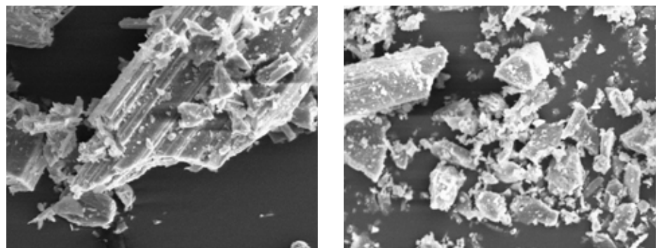
Abb. 9: REM-Aufnahmen von Alpha-Halbhydrat in einem handelsüblichen Fließestrich
